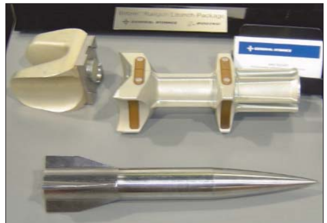
12. ábra. A Railgun nagysebességű lövedéke (Amaczi Viktor)
