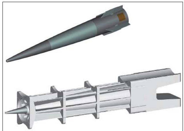
7. ábra. A HVP önállóan és a railgunhoz illeszkedő armatúrában [13]
